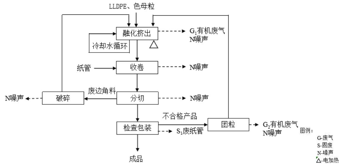
图 2-2 缠绕膜生产工艺流程图
