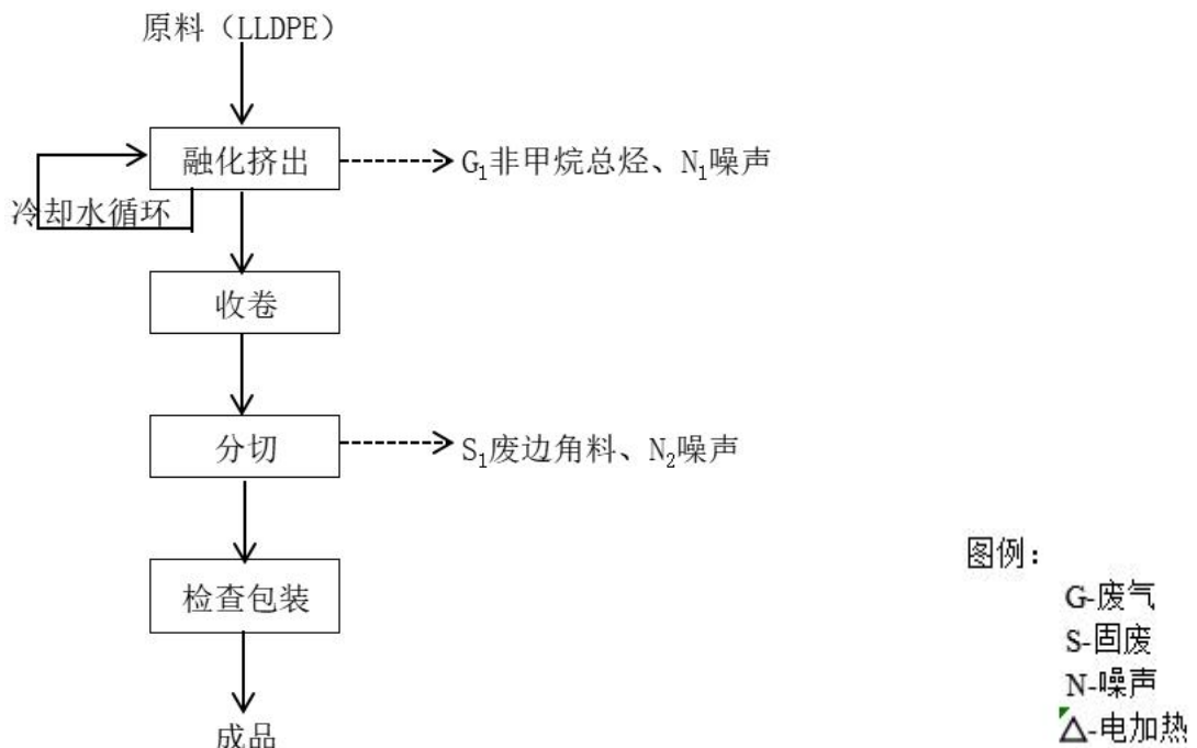
图 2-3 缠绕膜生产工艺流程图
