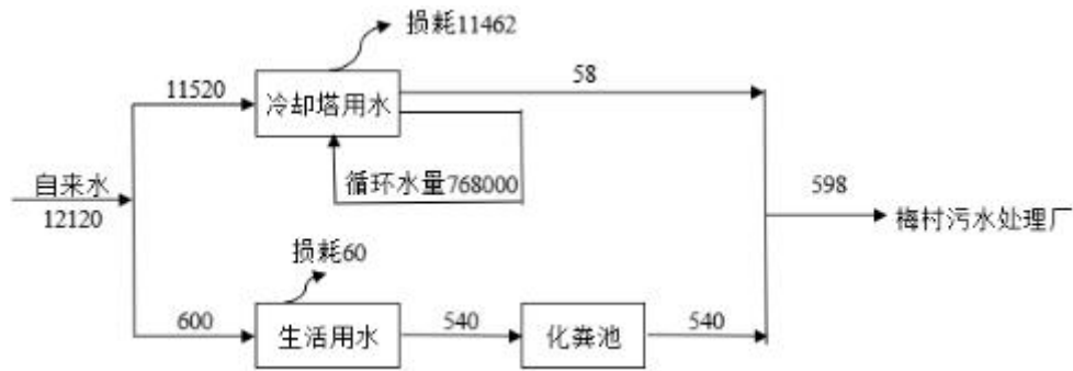
图 2-4 迁建前全厂核定水平衡图 单位：t/a
