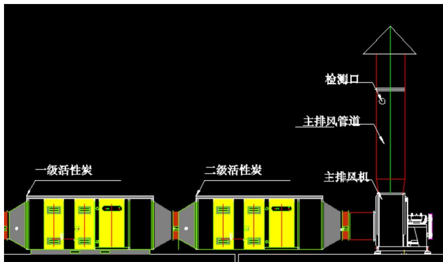
图 4-2 二级活性炭装置示意图
